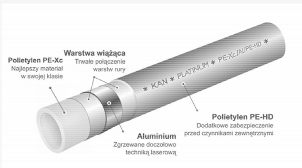
Konstrukcja rur PE-Xc/Al/PE-HD Platinum
